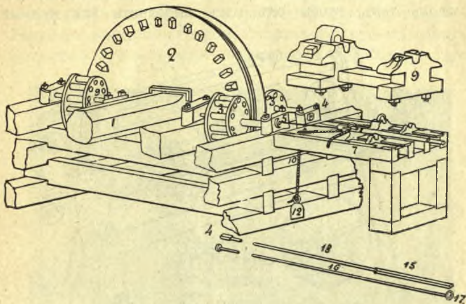
Станокъ времянь Петра I.
