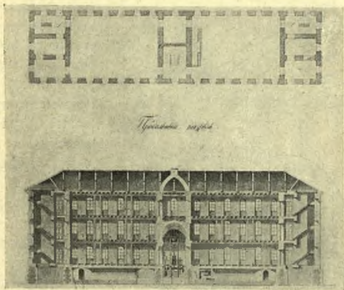
Корпусъ паровой машины.
