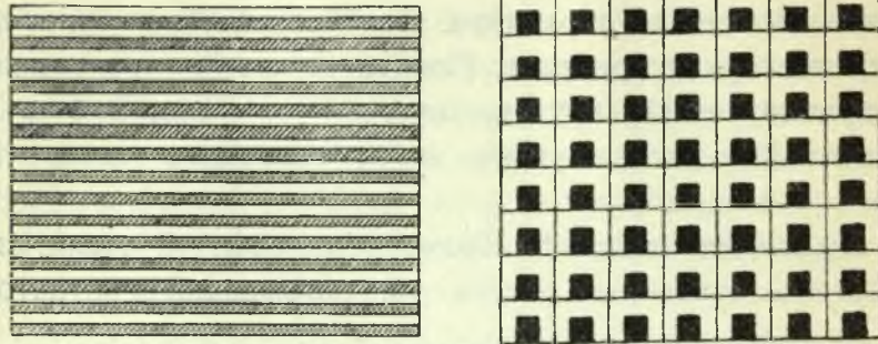
Пакеты изъ стали и желѣза для сварки дамасковыхъ полосъ.
