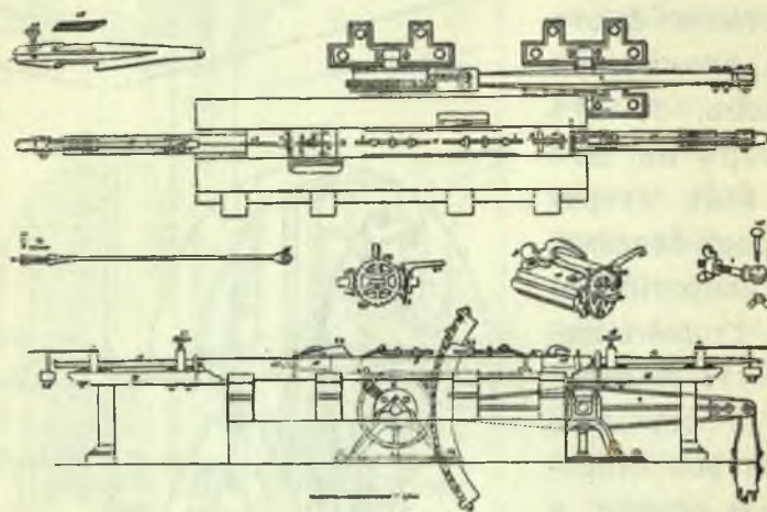
Шустовальный станокъ.
