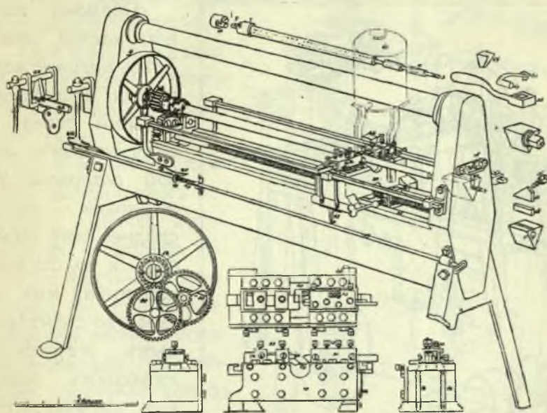
Токарный станокъ.
